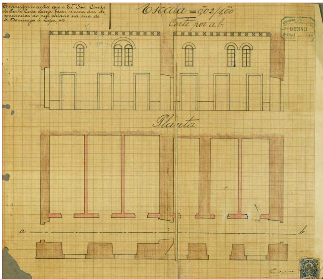
Figura 2 Planta referente a uma intervenção realizada em 1907, por um dos últimos descendentes do barão de Porto Côvo. AML, Obra : 4525, proc. n.º 3243/1.ª REP/PG/1907, p. 2.
