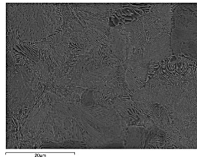
Fig. 10 - Microestrutura do aço, em secção transversal, revelada com nital a 2%, observada em MEV a 2200x.
