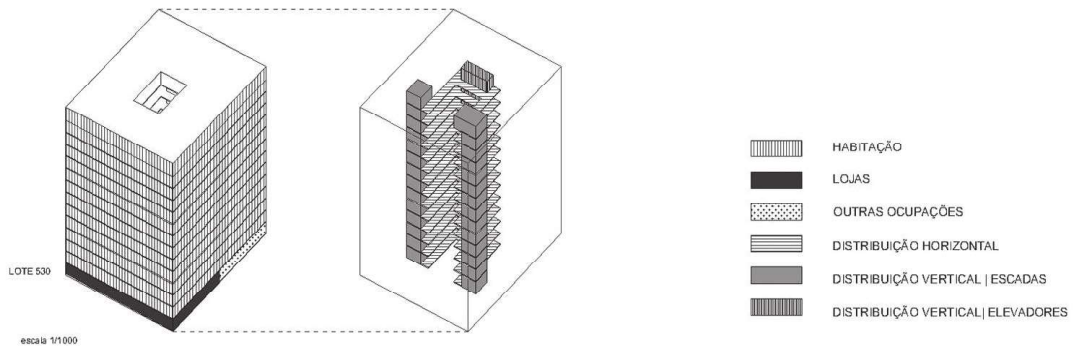
Figura 6 ▸ Estrutura em torre. Bairro do Condado, Zona J, Marvila, Lisboa
