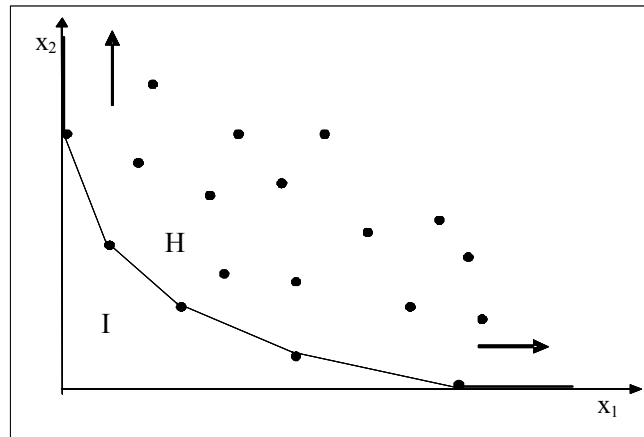
Figura 7 – Região H, domínio das variáveis ajustadas
