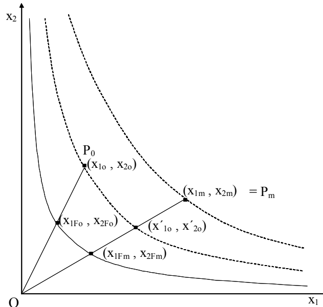
Figura 6 – Posicionamento das Curvas de Indiferença
