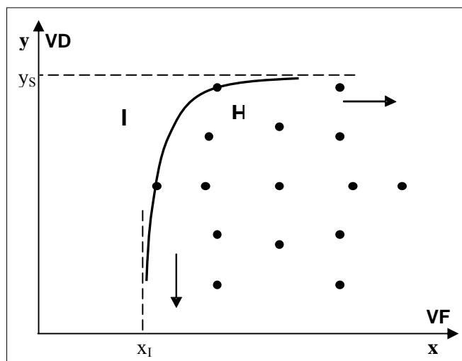
Figura 1 – Região H, domínio das variáveis
