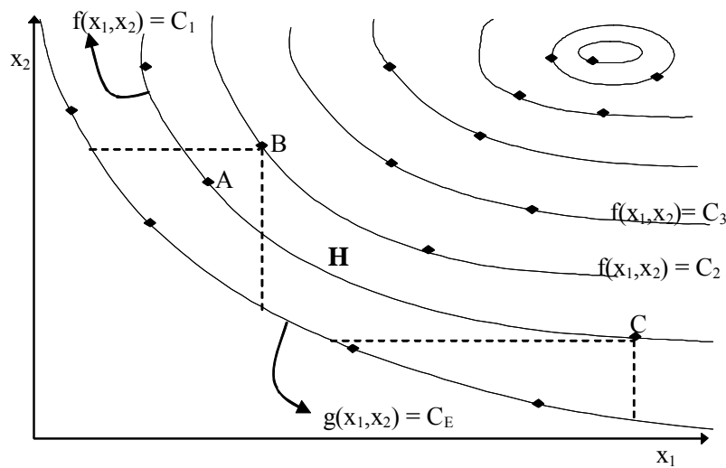
Figura 3 – Domínio da fdp da conjunta f(x_1, x_2)
