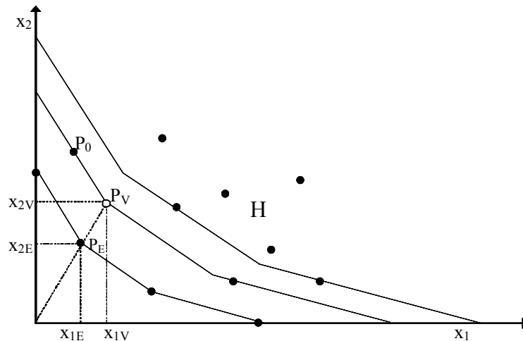
Figura 8 – Poligonais de indiferença
