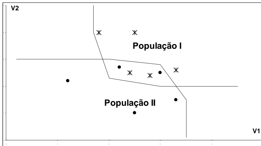
Figura 9 – Distribuição de duas Populações. Variáveis não ajustadas
