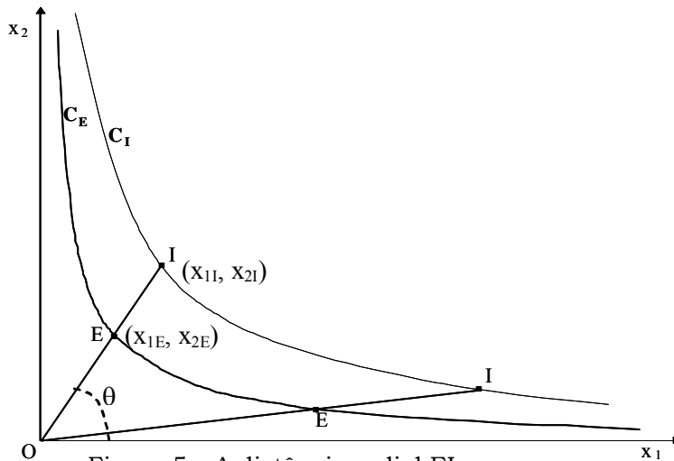
Figura 5 – A distância radial EI
