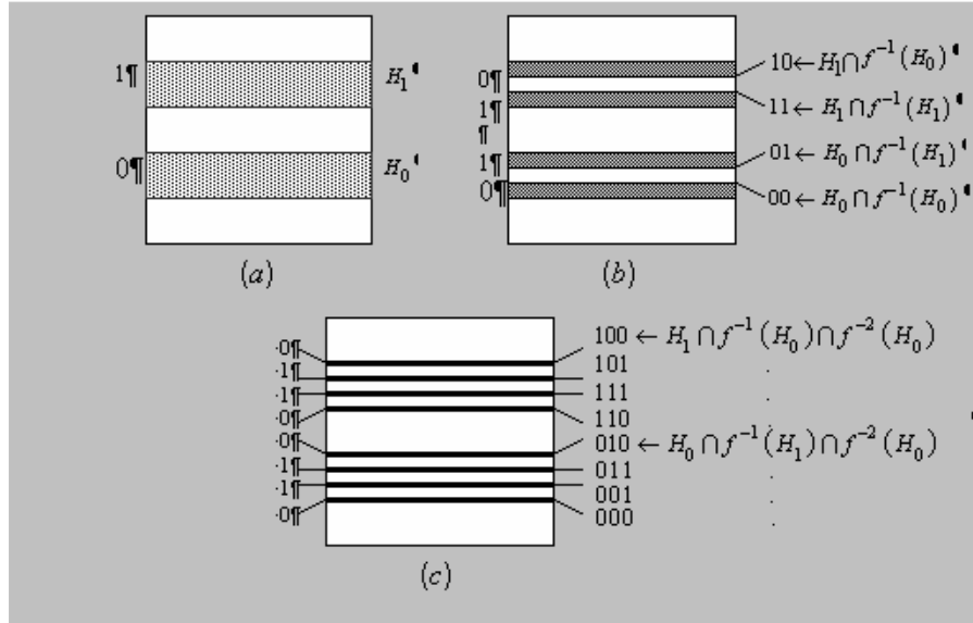
Figura 3.2. Codificação das faixas em f^{-i}(N) \cap Q , para: (a) i = 0 , (b) i = 1 ; (c) i = 2 .
